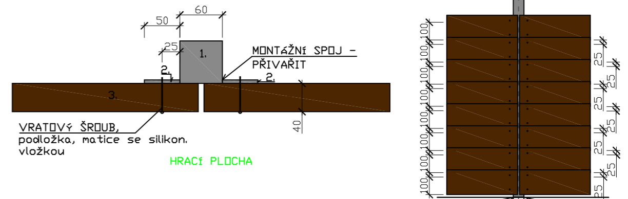
DETAILY UCHYCENÍ FOŠEN OHRAZENÍ NA SLOUPEK - ROHY
