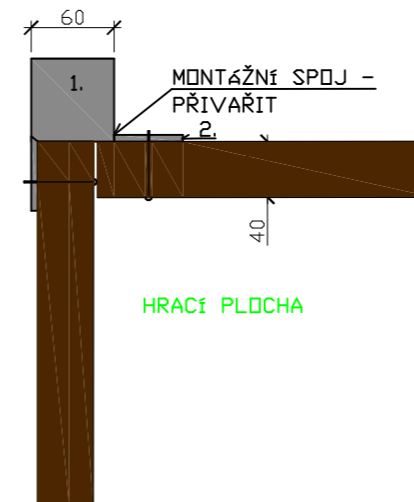
DETAILY UCHYCENÍ FOŠEN OHRAZENÍ NA SLOUPEK - ROHY
