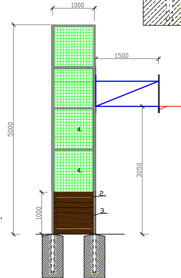
OHRAZENÍ - výklenek pro branku na házenou s konstrukcí na streetbasketbal
