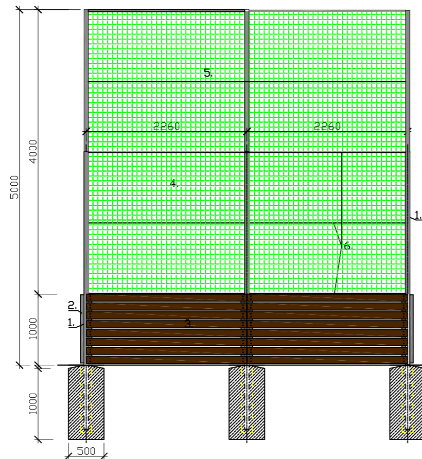
OHRAZENÍ - delší strany, dřevěné fošny, tkaná síť do v. 4,0m
