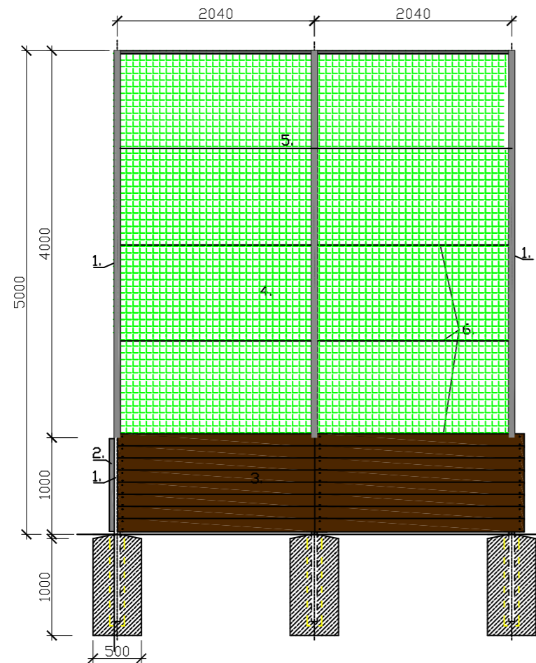
OHRAZENÍ - kratší strany, dřevěné fošny, tkaná síť do v. 4,0m
